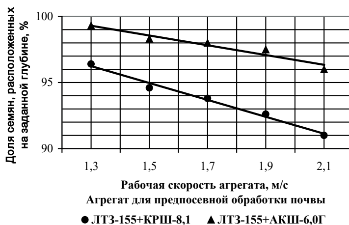
Рисунок 2 – Распределение семян сахарной свеклы на установленной глубине заделки после предпосевной обработки почвы агрегатами ЛТЗ-155+КРШ-8,1Г и ЛТЗ-155+ АКШ-6Г
